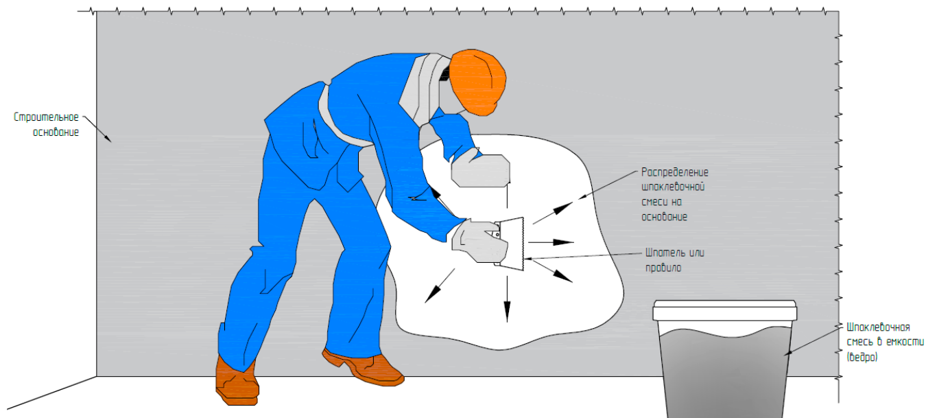
Рис. 14. Организация работ по нанесению шпаклевочной смеси
