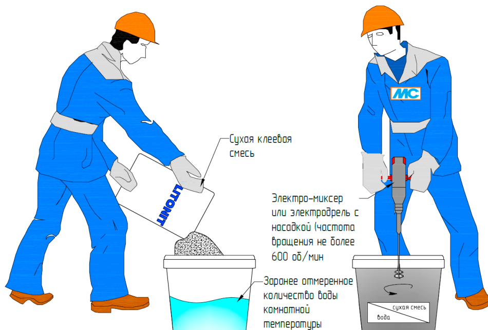
Рис. 15. Организация работ по затворению сухой клеевой смеси
